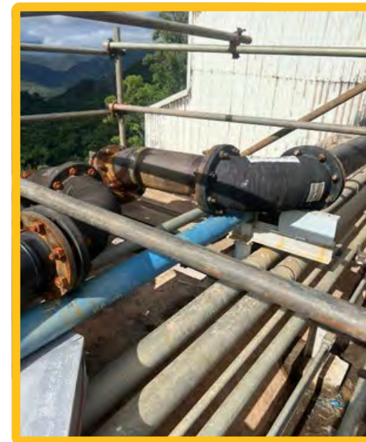
SUPORTAÇÃO DAS LINHAS DE RECALQUE DAS BOMBAS, MONTAGEM DA PLATAFORMA DO TQ-091, MONTAGEM DAS LINHAS DOS DRENOS DA CALHA DO MATEC E ADEQUAÇÃO DA LINHA DE RECALQUE DAS BOMBAS
