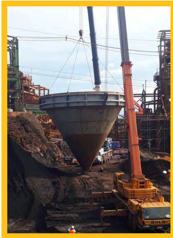
MONTAGEM DE ESPESSADORES - MINA DO PAU BRANCO - ITABIRITO/MG
