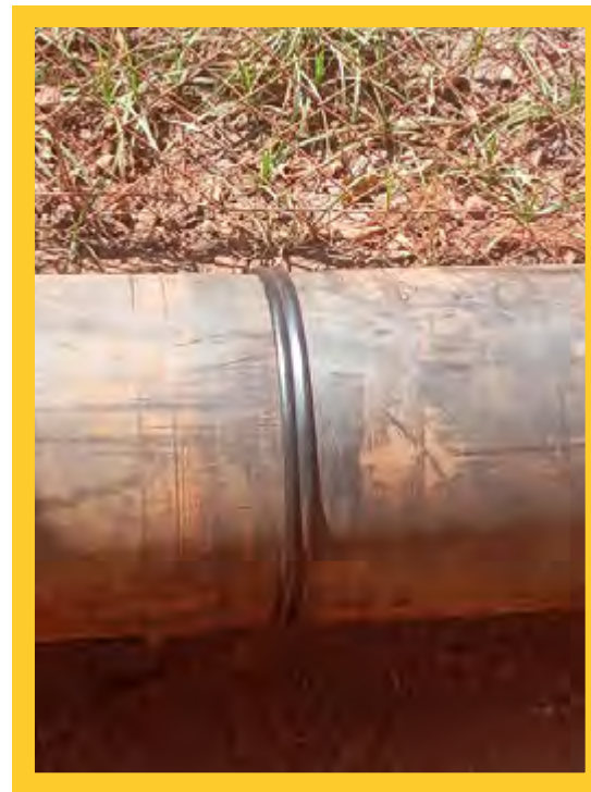
TRANSIÇÃO DE SOLDA DE TUBULAÇÃO DE AÇO CARBONO PARA PEAD - SUMP 3 - MINA DE CAUÊ - ITABIRA/MG
