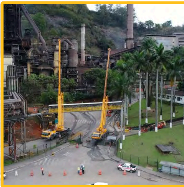
FABRICAÇÃO E MONTAGEM DE PASSARELA DE ACESSO - USINA MONLEVADE / MG
